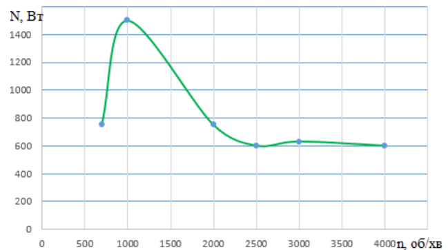
Рис. 5. Зміна витрат потужності на привід генератора 1601.3701
